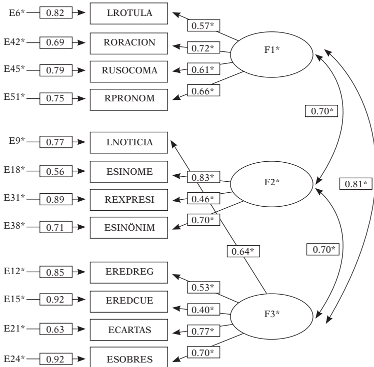
Figura X: EQS 6 aflengua 3factores resultante afe Chi Sq. =63.43 P=0.11 CFI=0.97 RMSEA=0.04
