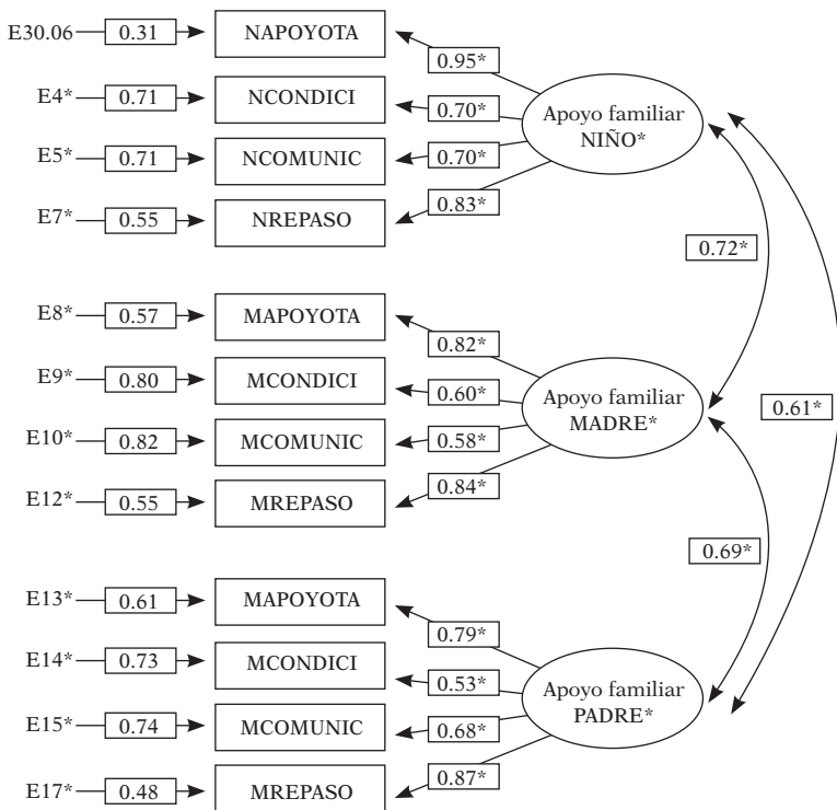
Figura X: EQS 6 sólo apofam tres_2 resultante Chi Sq. =130.88 P=0.00 CFI=0.91 RMSEA=0.16
